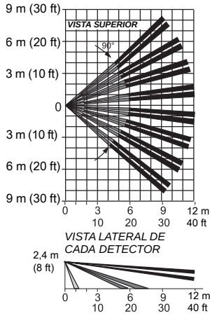
Figura 6: Patrón de la cubierta
